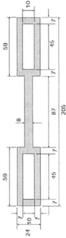
Diseño y dimensiones de la contra asa:
