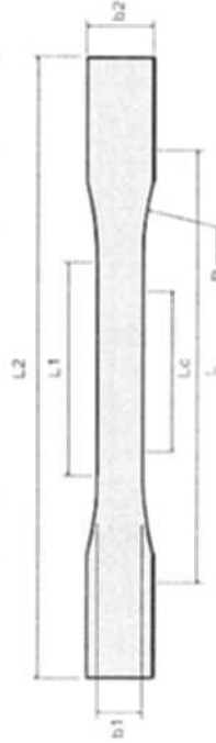
Especimen de ensayo: Tipo I moldeado con el compuesto plástico que se solicita en la producción de la asa.
